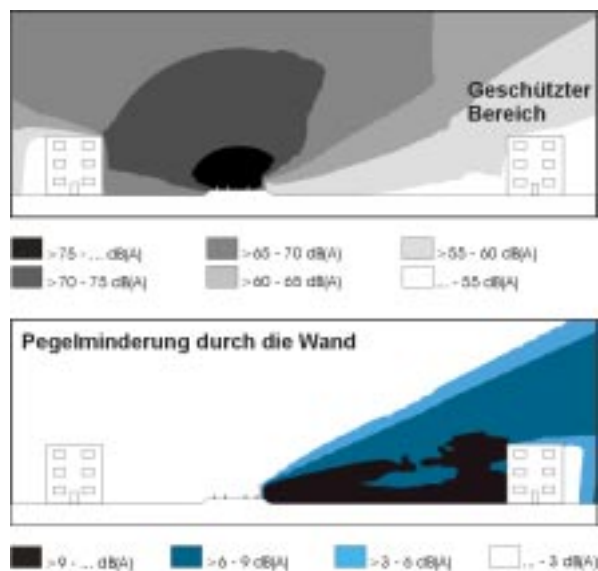
Abbildung 5: Schallschutzwand (einseitig)
