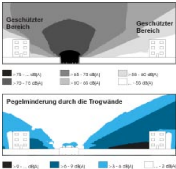
Abbildung 10: Trog
